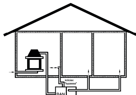
Ventilátor s bypassem ve sklepe
