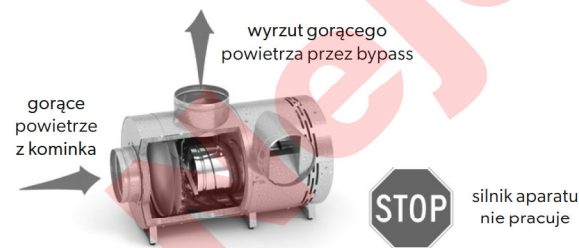
Rysunek 1.c. Aparat nie pracuje, np. brak prądu
