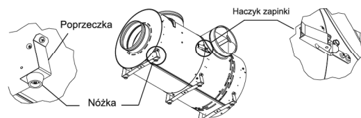
Rysunek 4.b. Budowa
