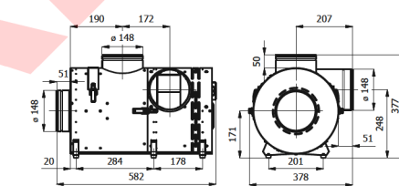
Rysunek 3.b. Wymiary BANANeco2-II
