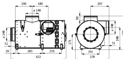
Fig 3.c. Dimensions BANANeco3-II
