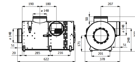
Rysunek 3.c. Wymiary BANANeco3-II
