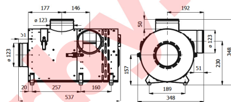
Rysunek 3.a. Wymiary BANANeco1-II
