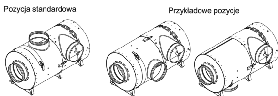
Rysunek 2. Pozycje pracy bypassa BANeco
