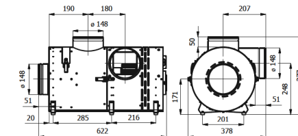
Fig 3.c. Dimensions BANANeco3-II
