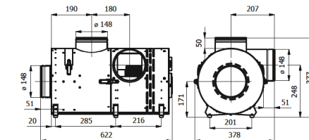
Rysunek 3.c. Wymiary BANANeco3-II
